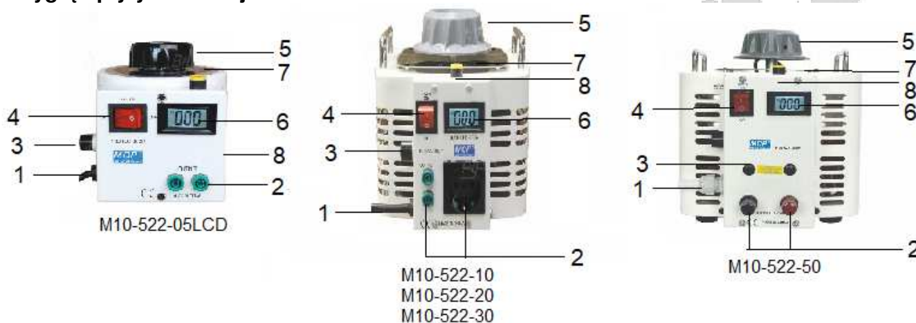
Wygląd płyty czołowej autotransformatora
