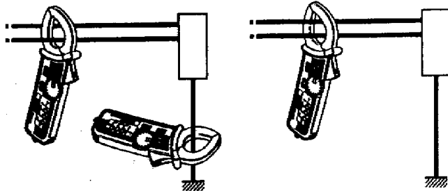
Rys. 1 Pomiar w typowym układzie
