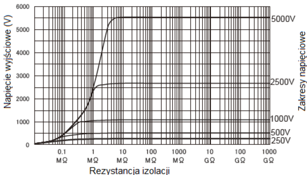
Charakterystyka wyjściowa KEW3125A/3025A
