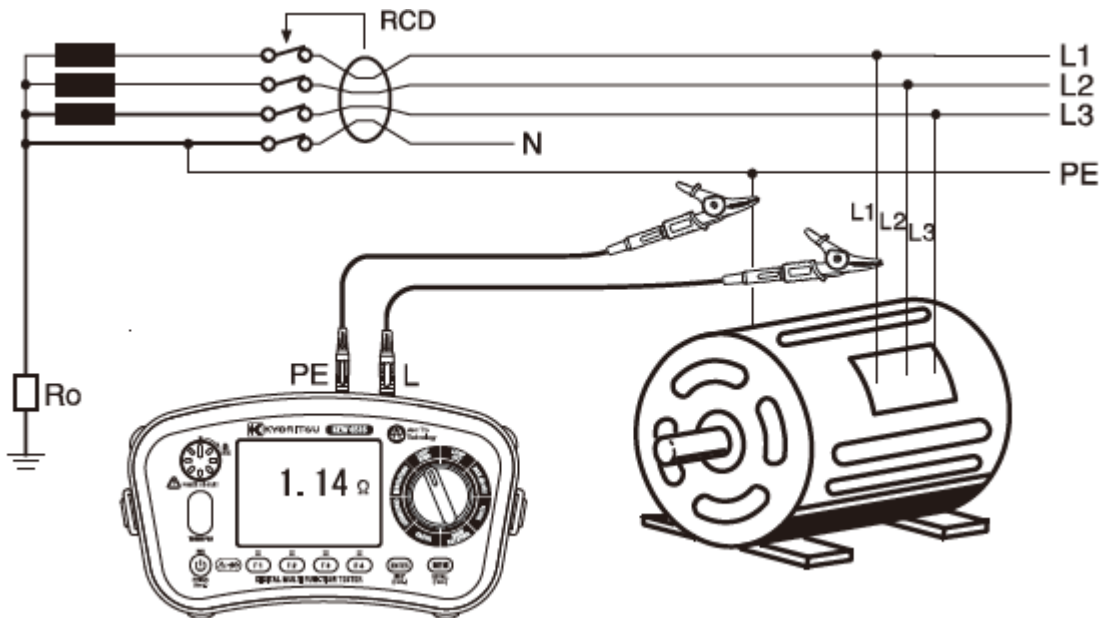
Pomiar 2-przewodowy L-PE
